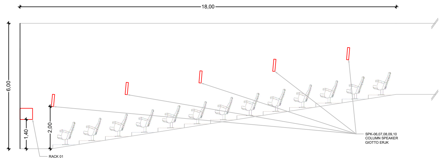
TOMH B-B'
