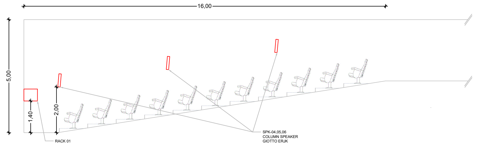
ΤΟΜΗ Β-Β'
