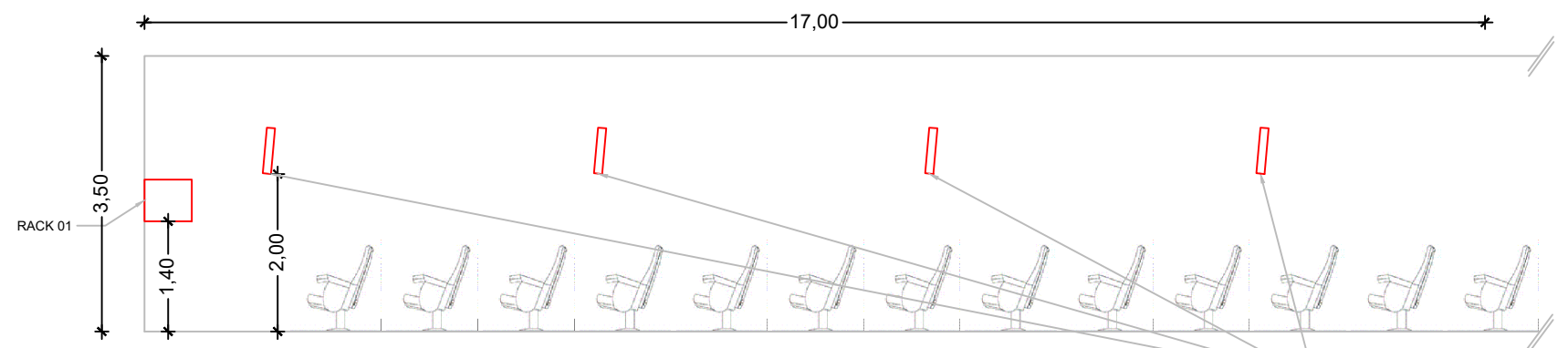
TOMH B-B'
