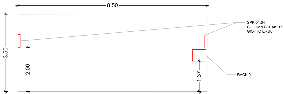
TOMH A-A'
