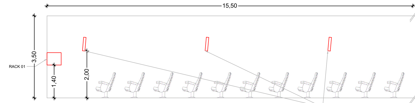
ΤΟΜΗ Β-Β'
